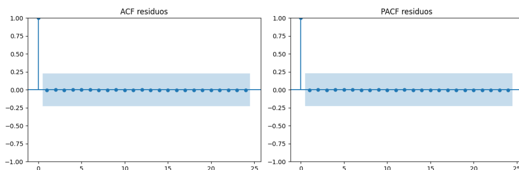
Figura 1: Diagnóstico de residuos del modelo ARIMA seleccionado
